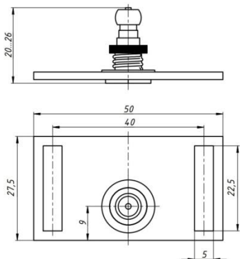
Рис. 3. Ригель Promix-AD.DB.13
