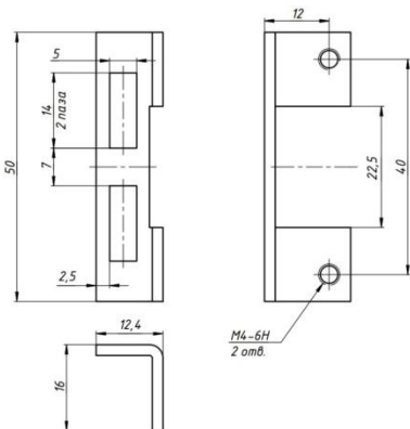
Рис. 5. Кронштейн Promix-AD.BR.06
