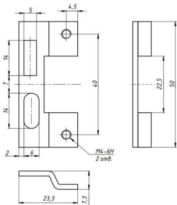
Рис. 4. Кронштейн Promix-AD.BR.05
